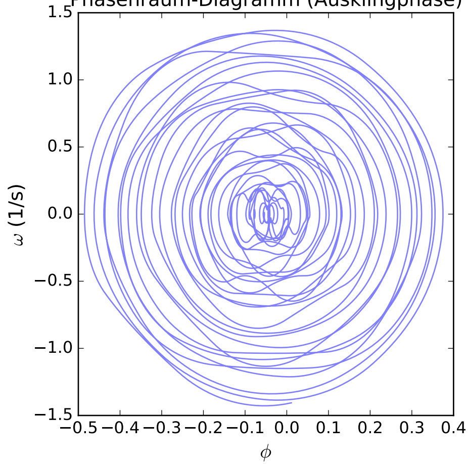
Phasenraum-Diagramm (Ausklingsphase)
